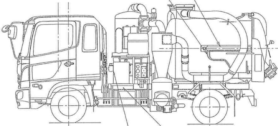
吸引ポンプ
